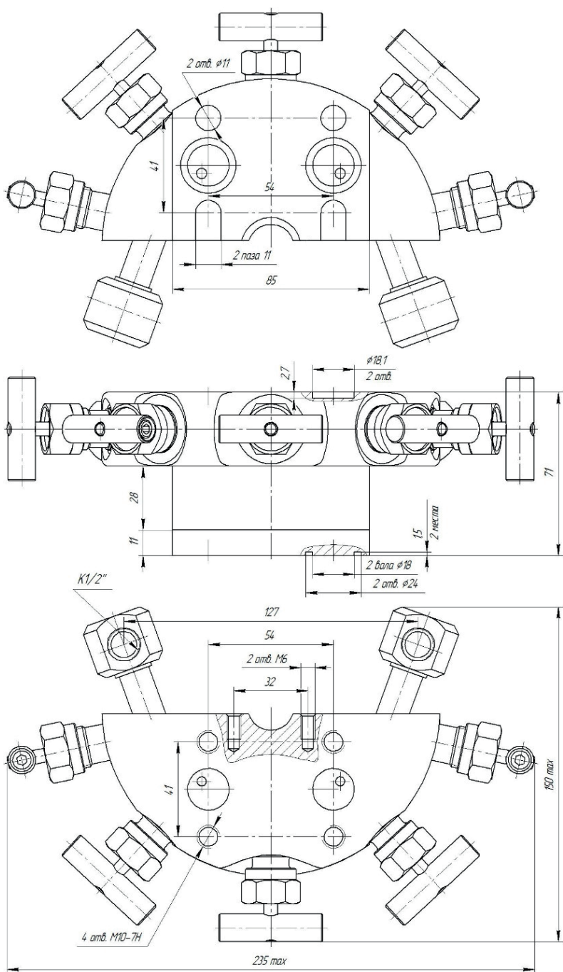
Рисунок А.17 — Блок клапанный БКН5-7-00
