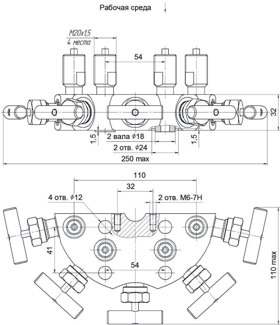
Рисунок А.20 — Блок клапанный БКН5-115-01
