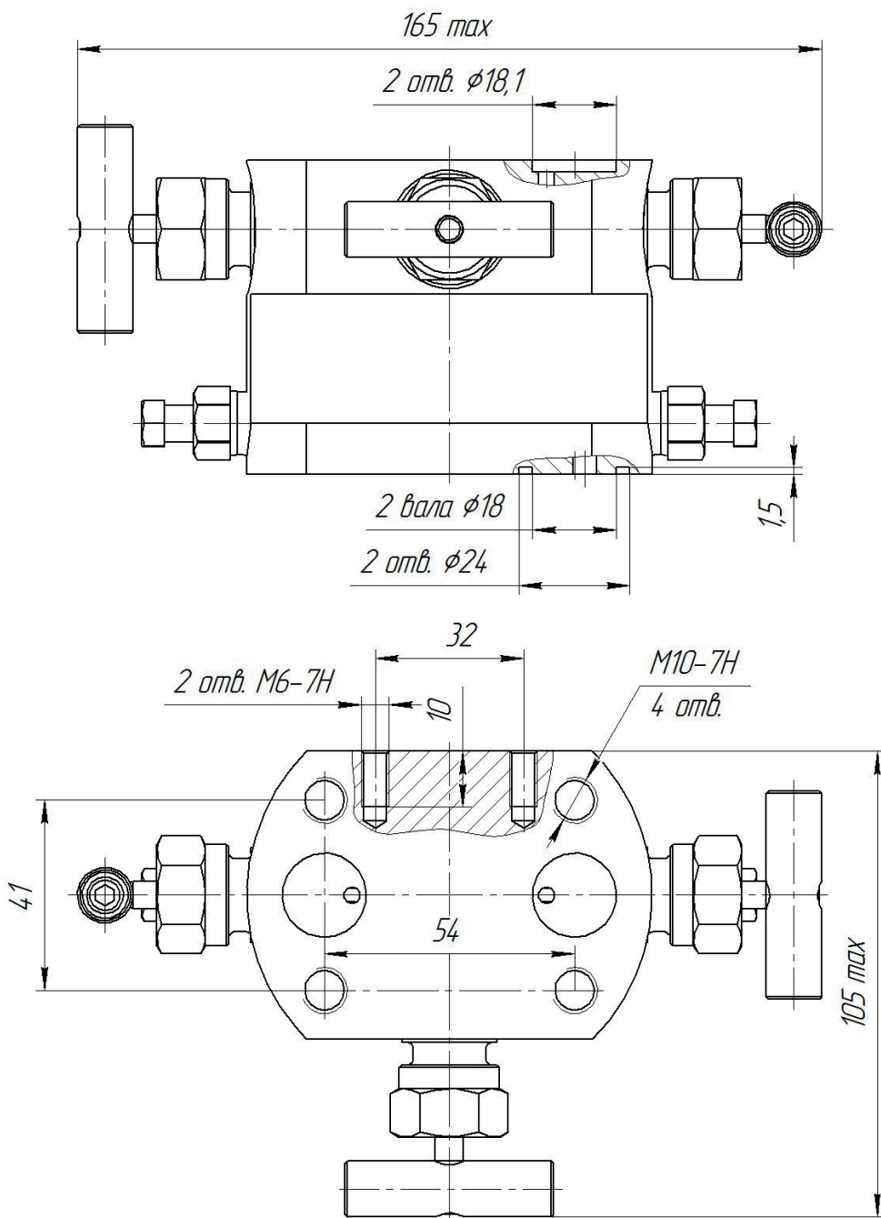
Рисунок А.4 — Блок клапанный БКНЗ-4-11
