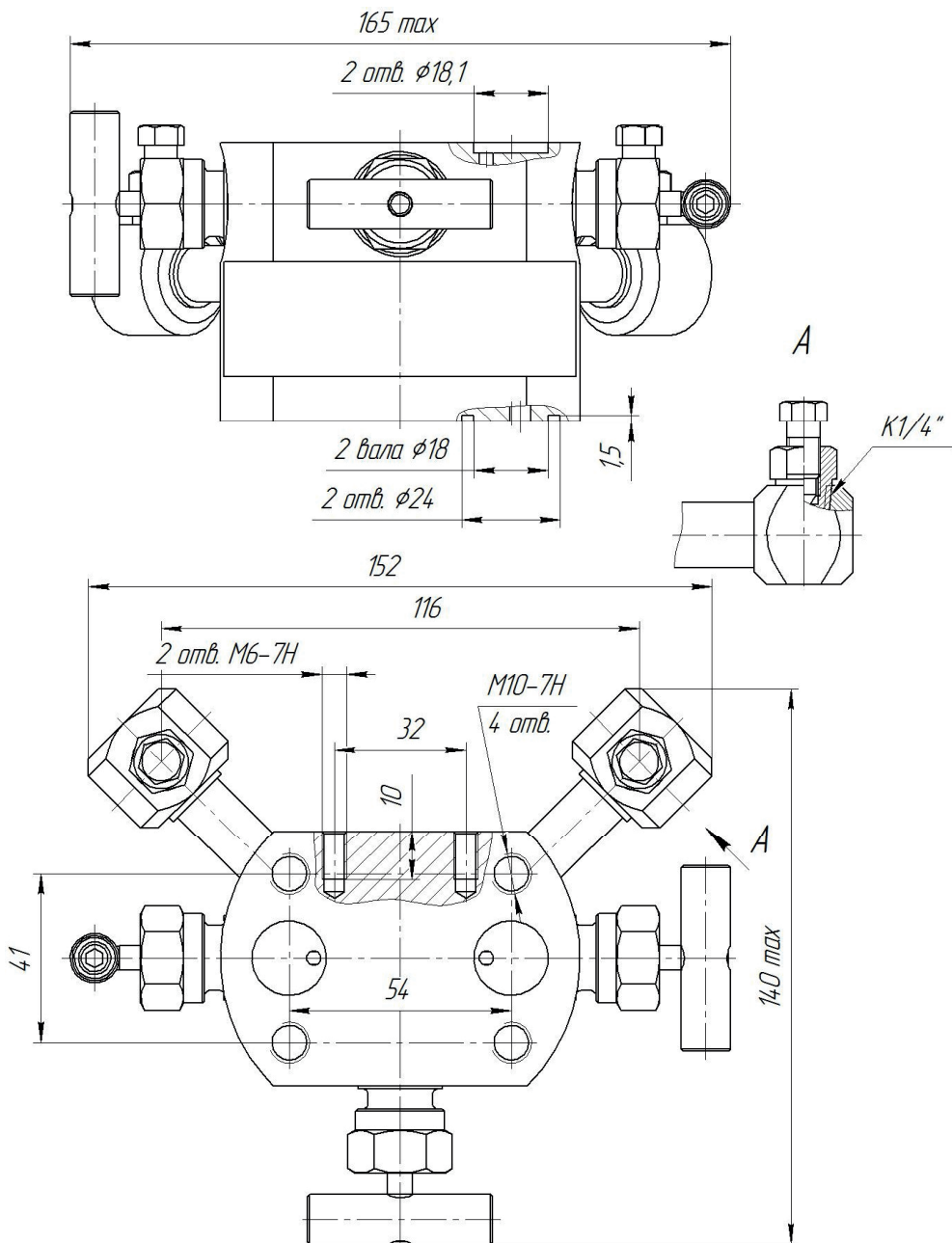
Рисунок А.3 — Блок клапанный БКНЗ-4-10
