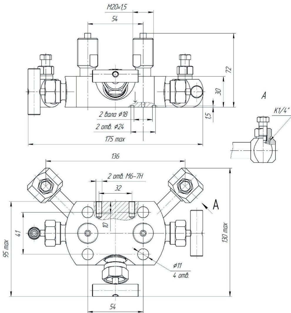
Рисунок А.9 — Блок клапанный БКН3-11-31
