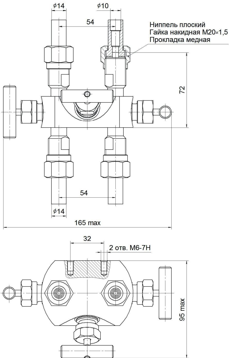
Рисунок А.12 — Блок клапанный БКН3-11-20П2
