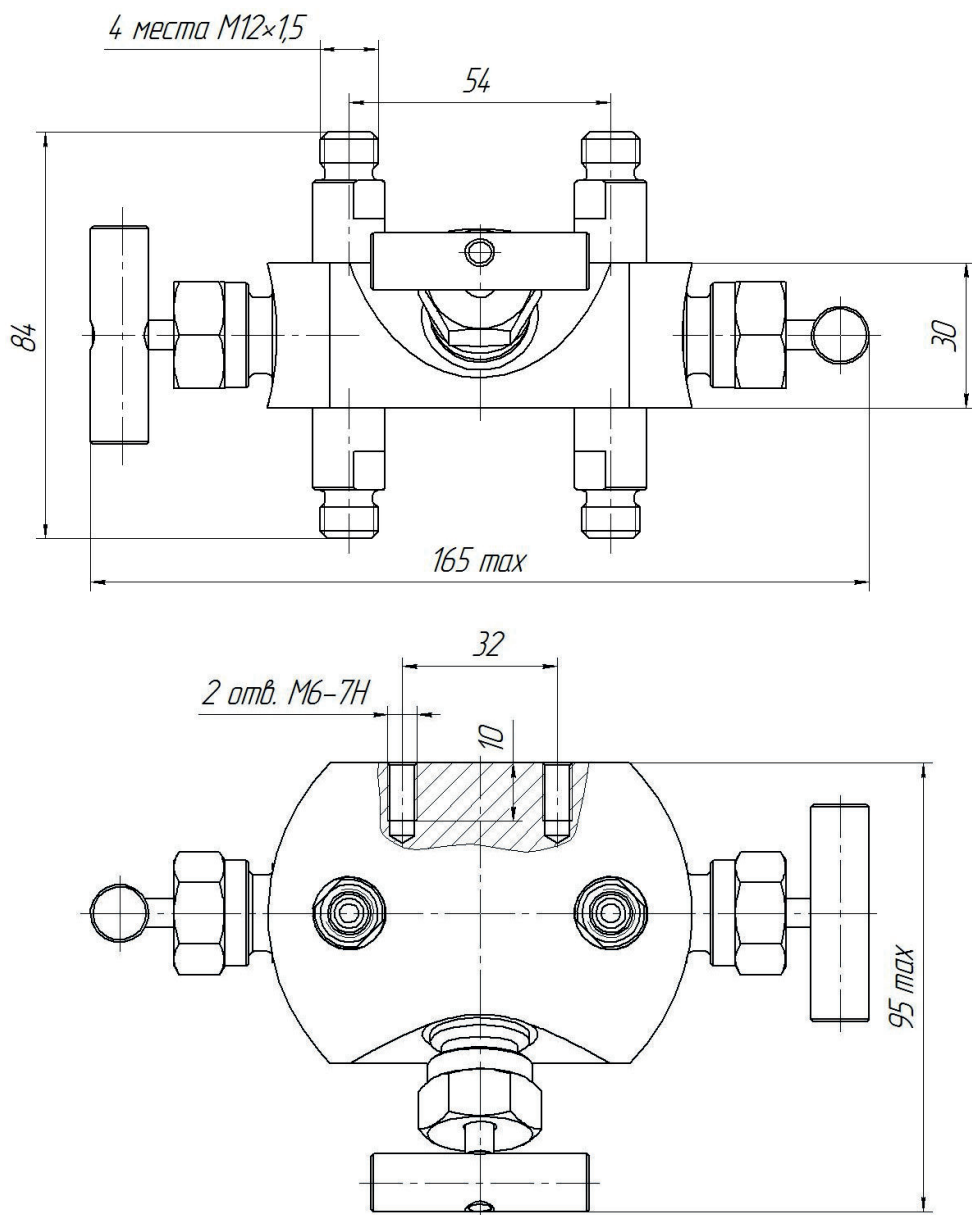
Рисунок А.11 — Блок клапанный БКН3-11-12С2
