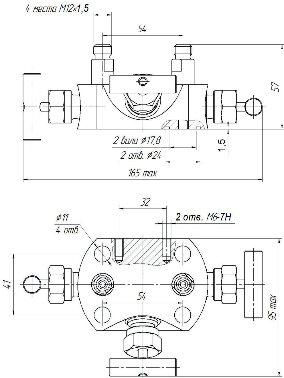
Рисунок А.10 — Блок клапанный БКНЗ-11-12С
