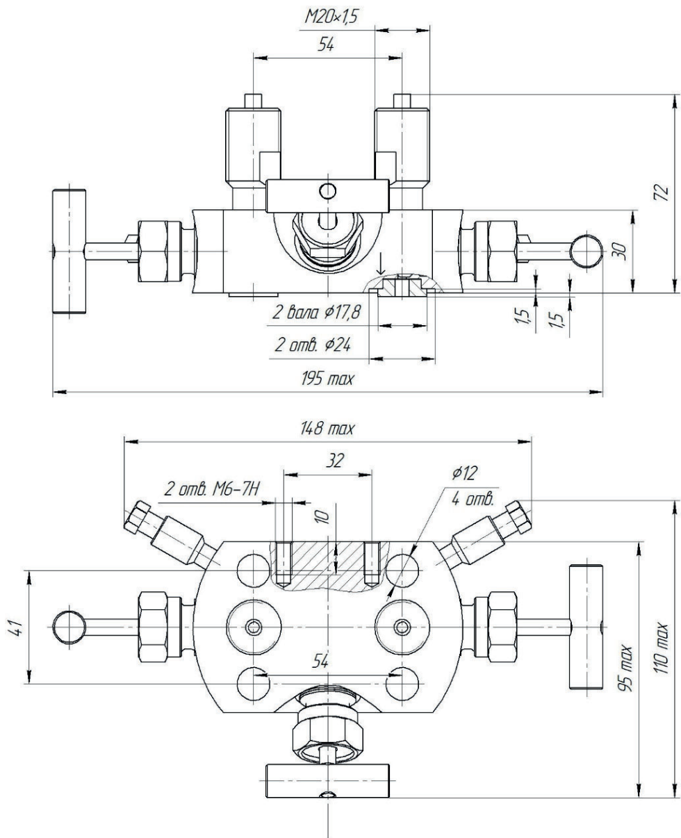
Рисунок А.15 — Блок клапанный БКНЗ-111-21
