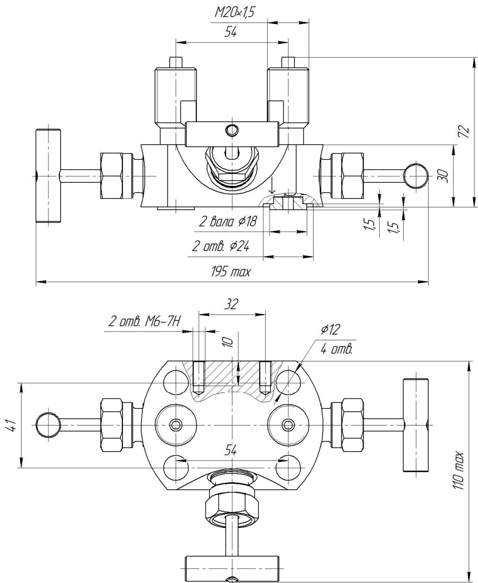
Рисунок А.13 — Блок клапанный БКНЗ-111
