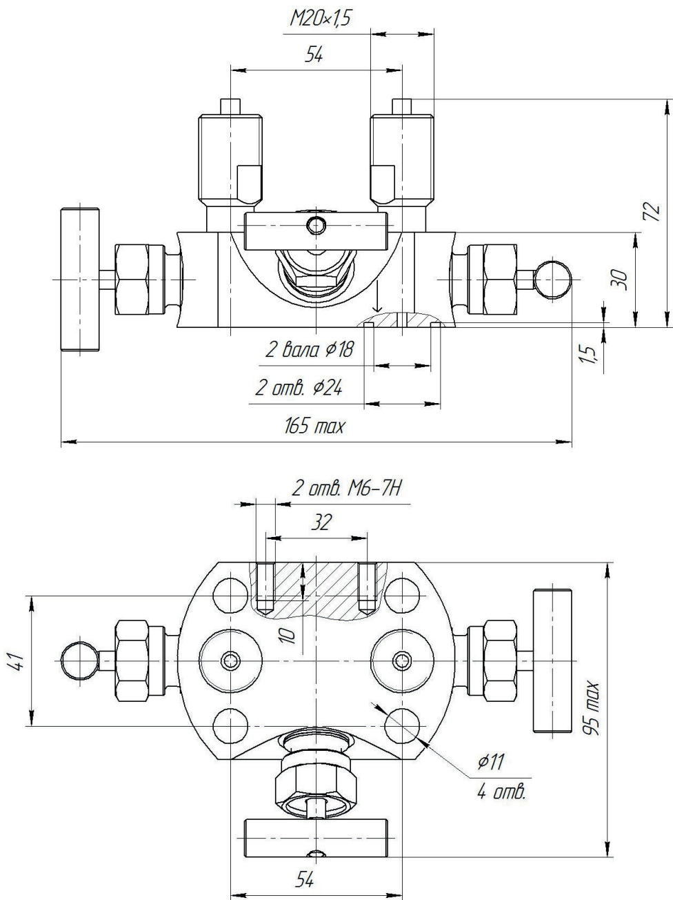
Рисунок А.5 — Блок клапанный БКНЗ-11
