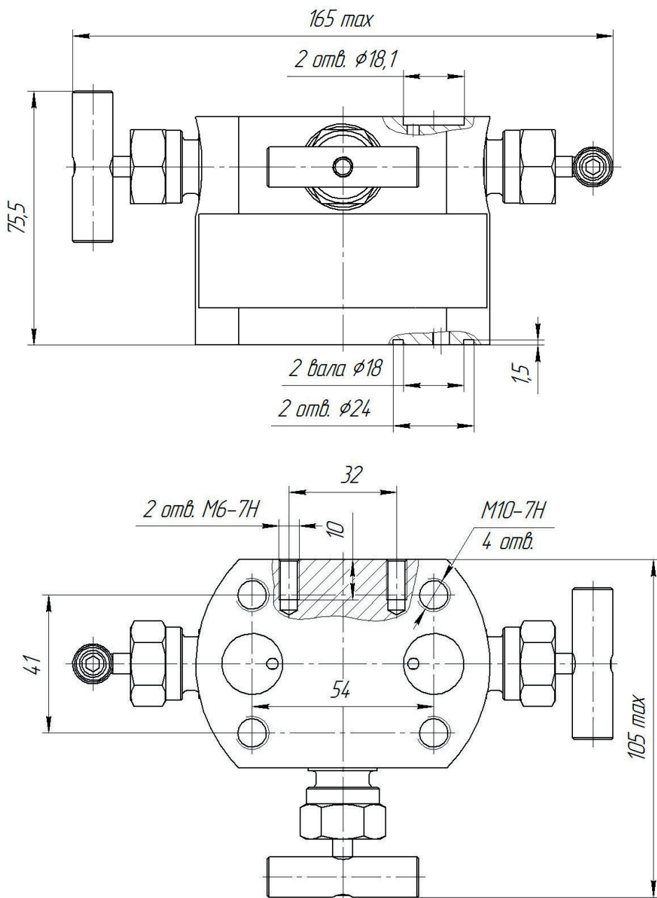
Рисунок А.1 — Блок клапанный БКНЗ
