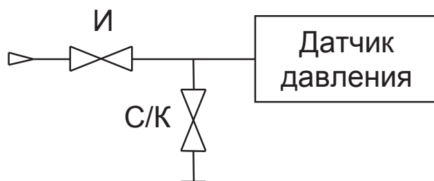
Рисунок А.2 – Клапанный блок БКН2
