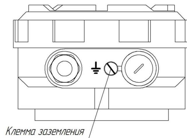
Рис. 5.2 Клемма заземления
