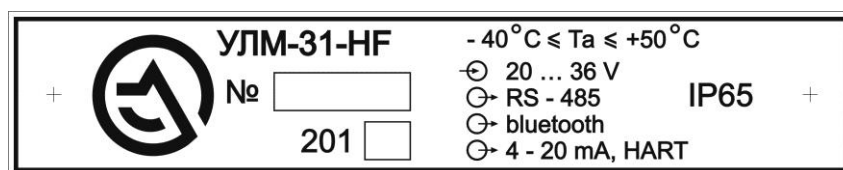
Рис. 3.5. Типовой шильдик УЛМ-31-HF
