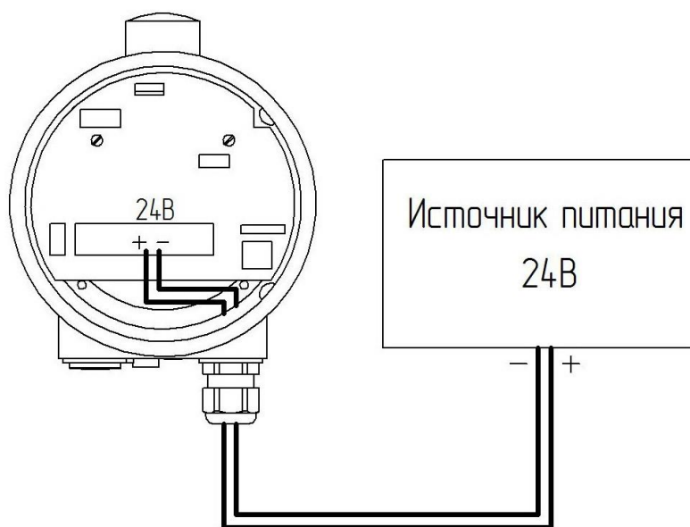
Рис. 5.5 Схема подключения уровнемера к ИП
