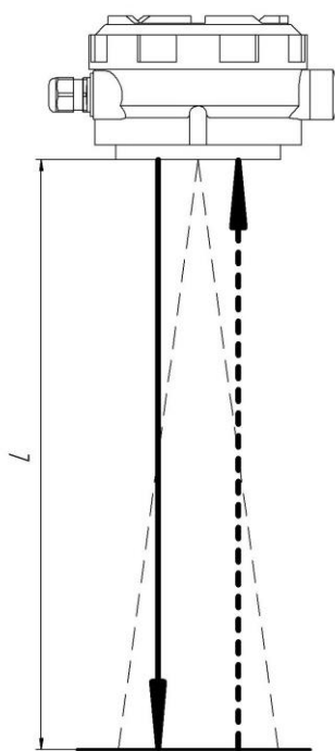
Рис. 3.10. Принцип измерения.
