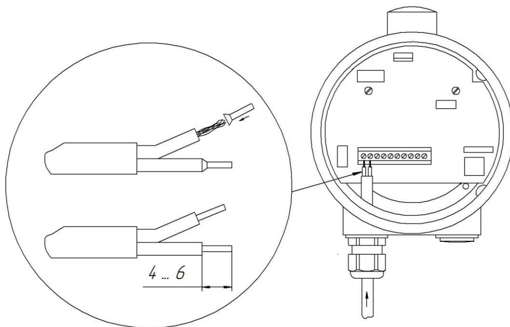
Рис. 5.8 Подключение уровнемера.
