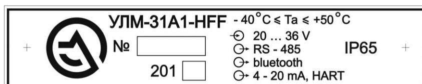
Рис. 3.8. Типовой шильдик УЛМ-31A1-HF-F
