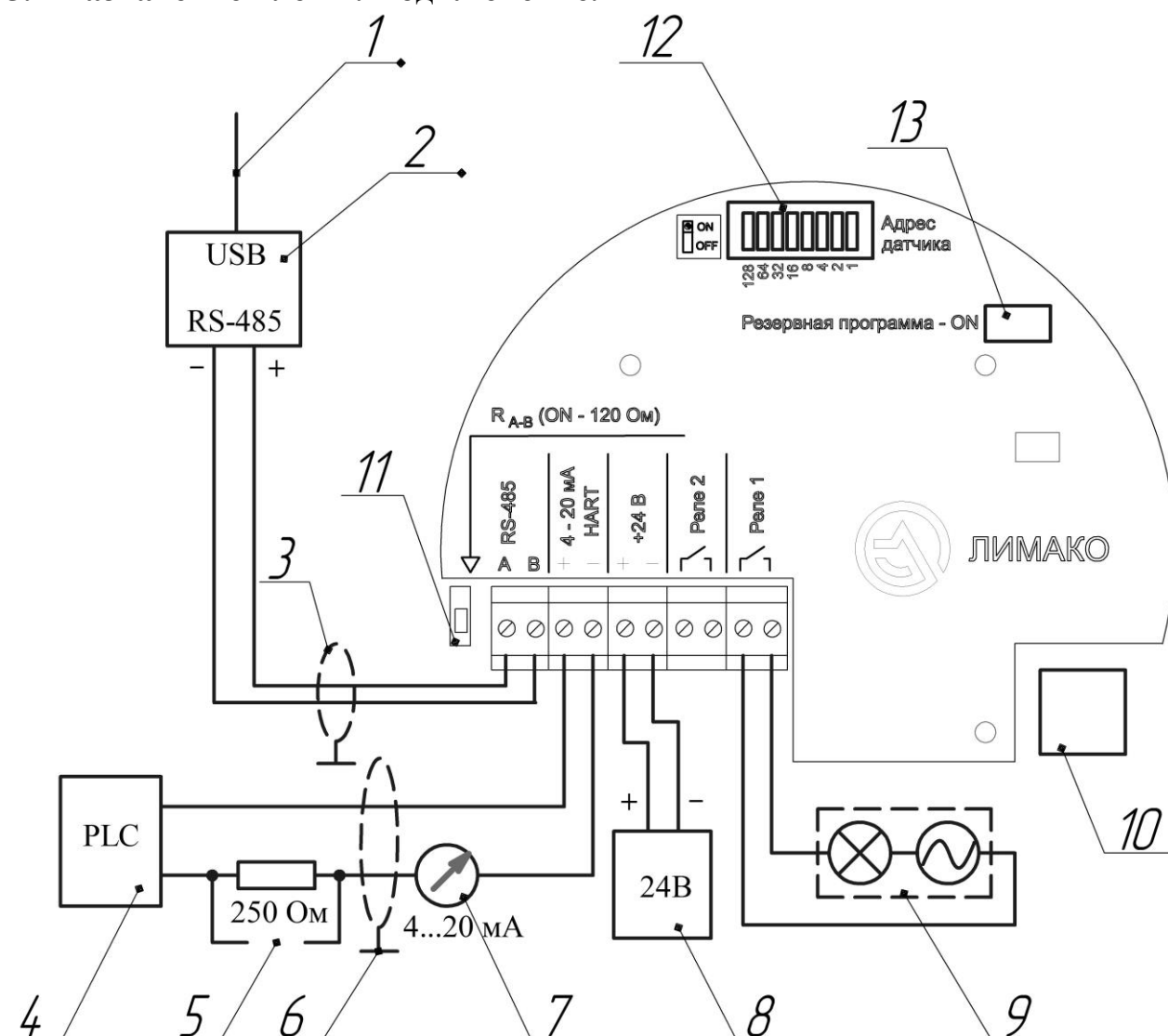
Рис. 5.3 Подключение уровнемеров УЛМ-31А1, УЛМ-31-НФ, УЛМ-31-НФ-Ф, УЛМ-31А1-НФ и УЛМ-31А1-НФ-Ф.
