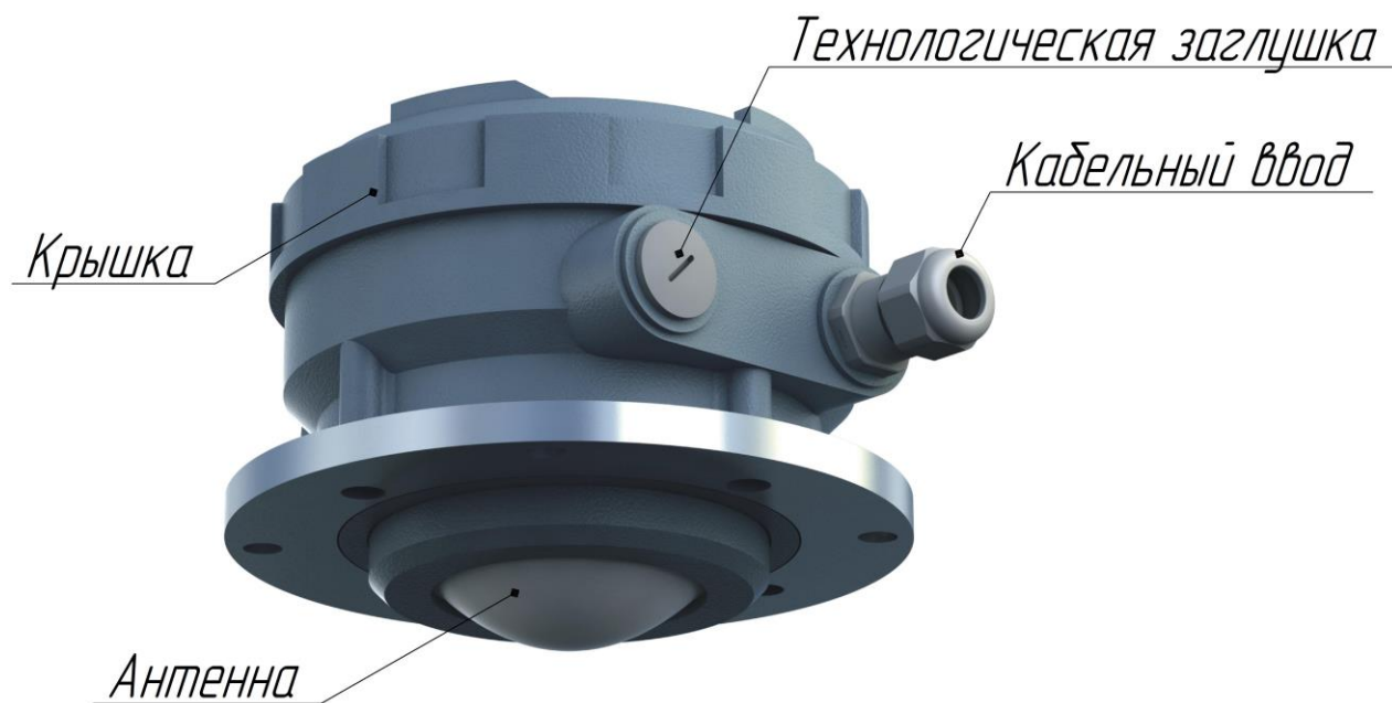
Рис. 3.1. Внешний вид и расположение основных элементов уровнемера УЛМ-31-НФ, УЛМ-31А1-НФ.
