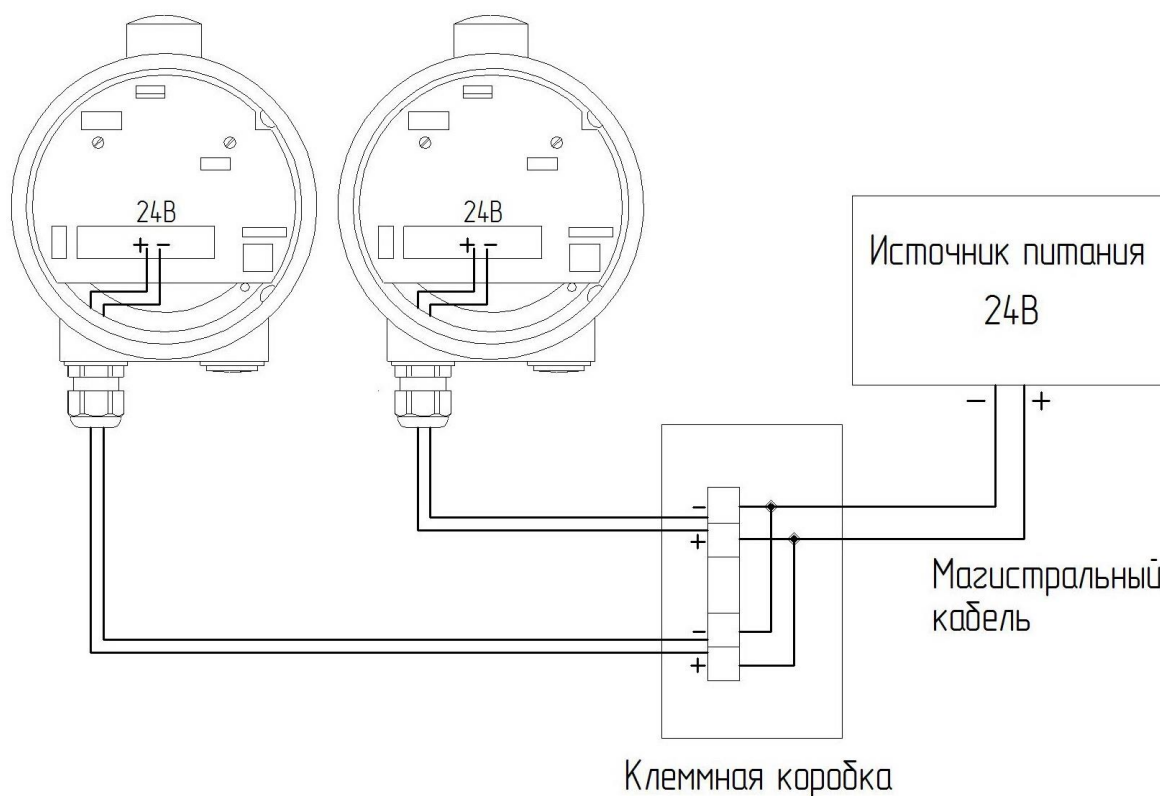
Рис. 5.6 Схема подключения уровнемеров к ИП с использованием клеммной коробки.
