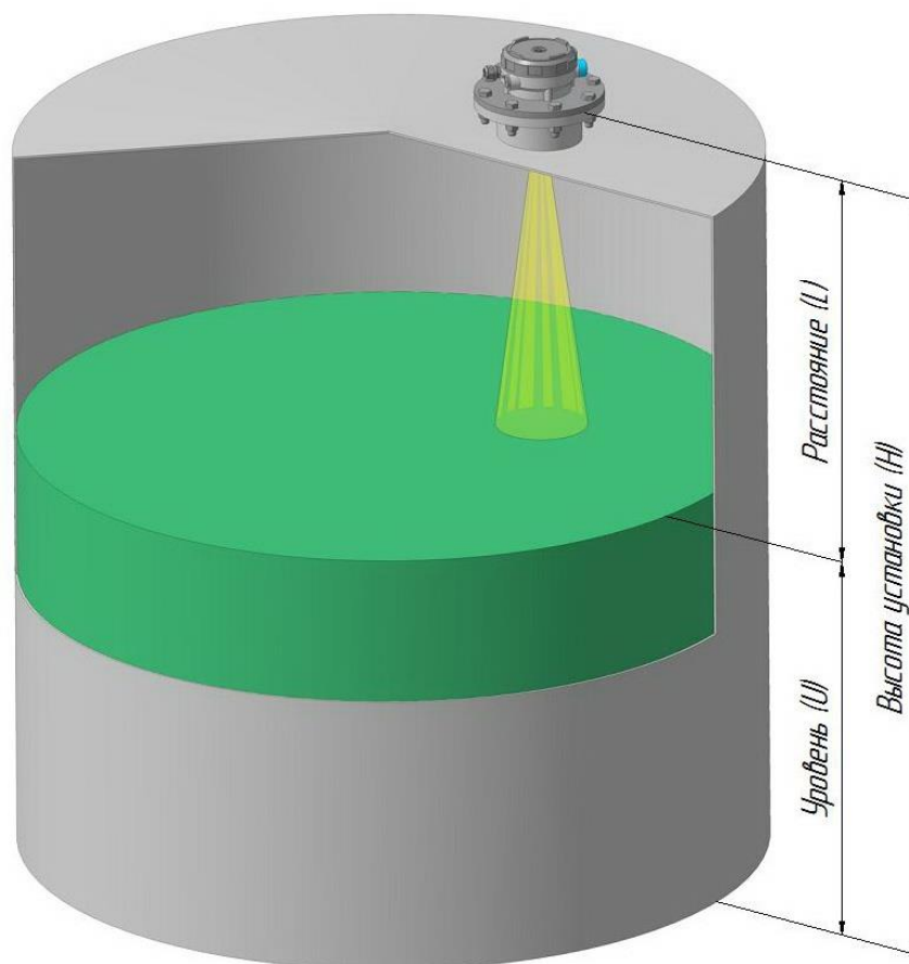
Рис. 3.9. Уровнемер на резервуаре.
