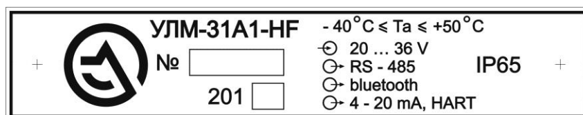
Рис. 3.7. Типовой шильдик УЛМ-31A1-HF
