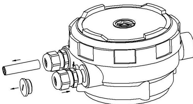
Рис. 5.7 Установка второго кабельного ввода
