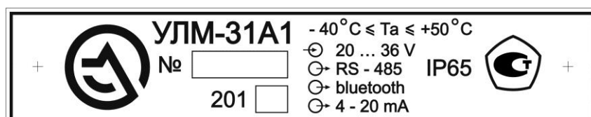
Рис. 3.6. Типовой шильдик УЛМ-31A1
