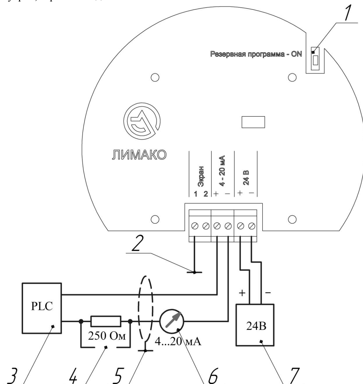
Рис. 5.4 Подключение уровнемера модификации УЛМ-31А1-НF-F-LC.
