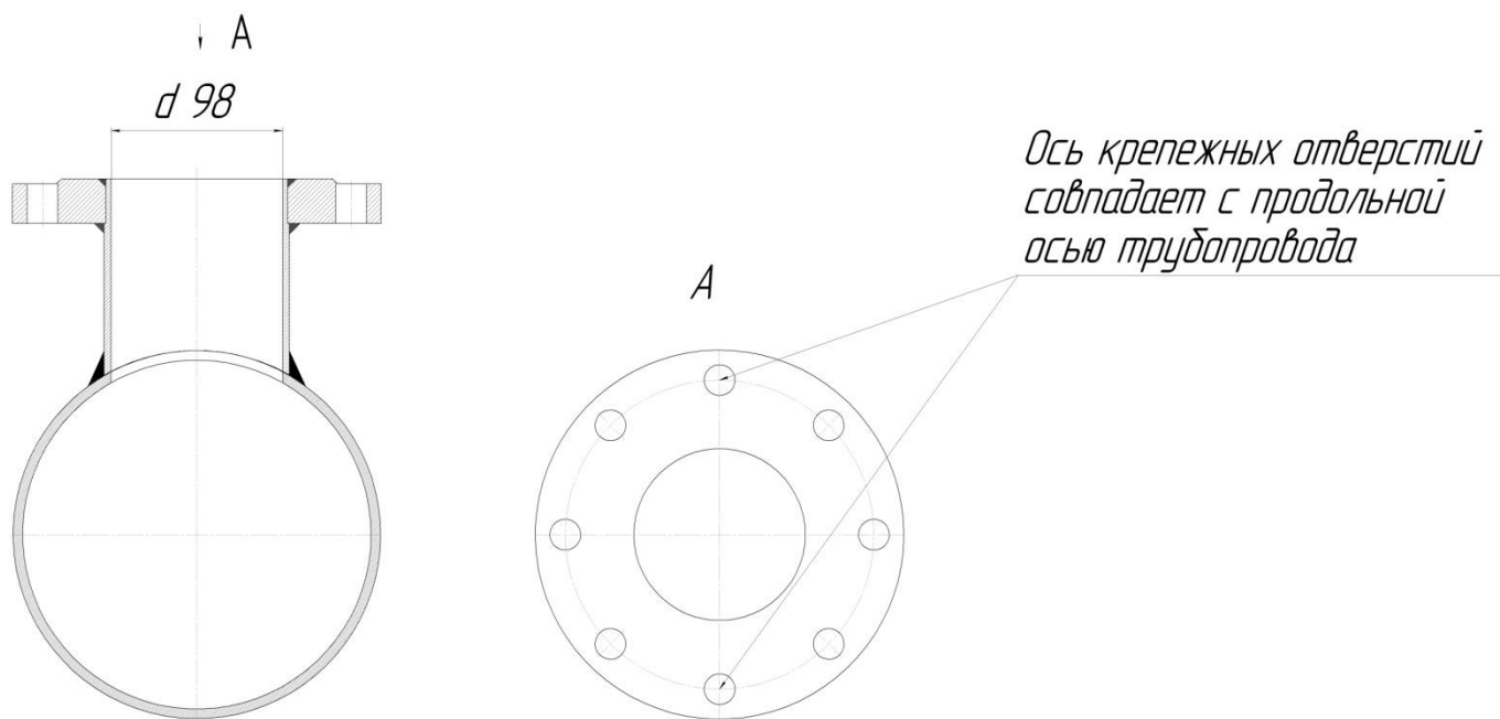
Рис.Д12 Монтаж патрубка приварного из состава КМЧ
