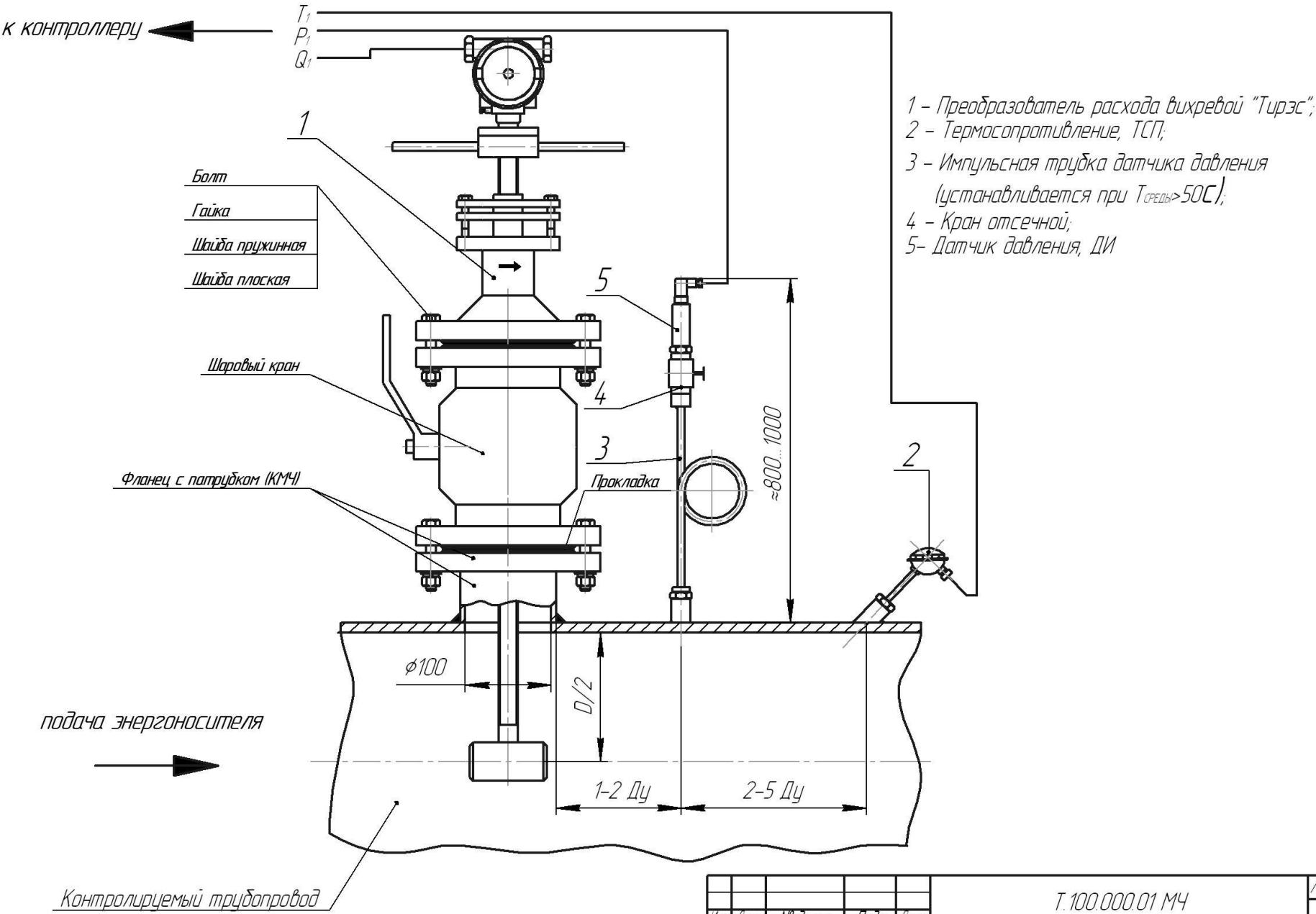
Рис. 5 Установка преобразователя расхода (исполнение С2) на трубопроводе
